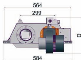
Поперечный разрез
